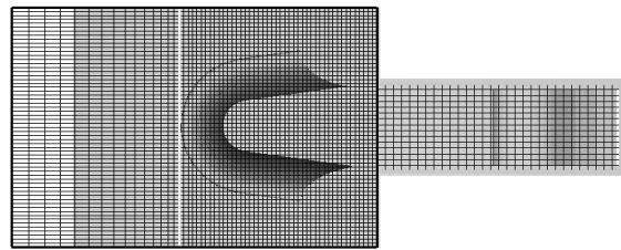
ب) شبکه بندی در پلان
