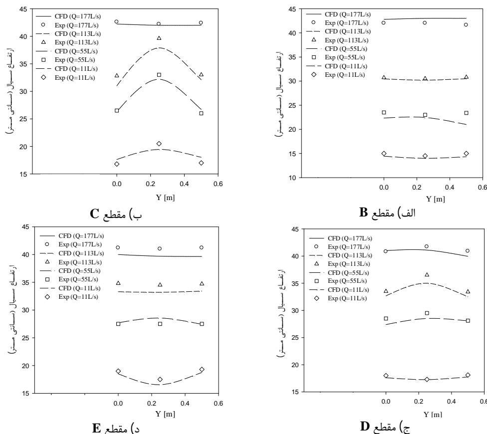
شکل 6 مقایسه عمق جریان در مقاطع عرضی بین داده‌های آزمایشگاهی و نتایج عددی (مؤسسه تحقیقات آب وزارت نیرو، 1375)
